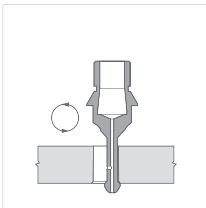
3_Escareação inferior
