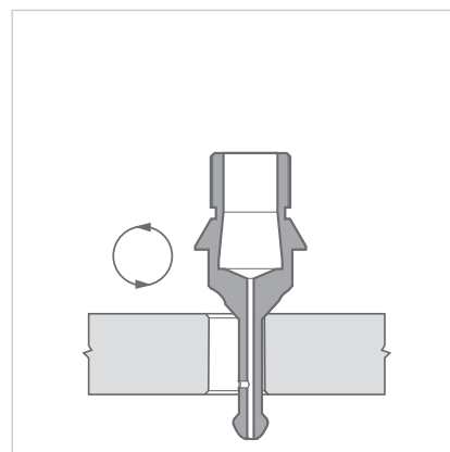
4_Escareação superior
